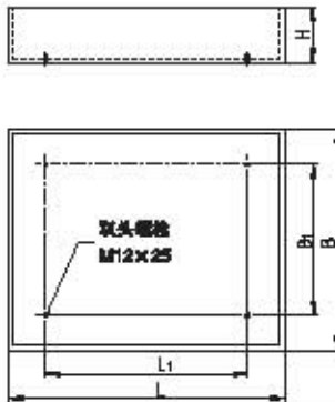
无底脚的集油槽
