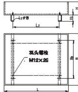
有底脚的集油槽
