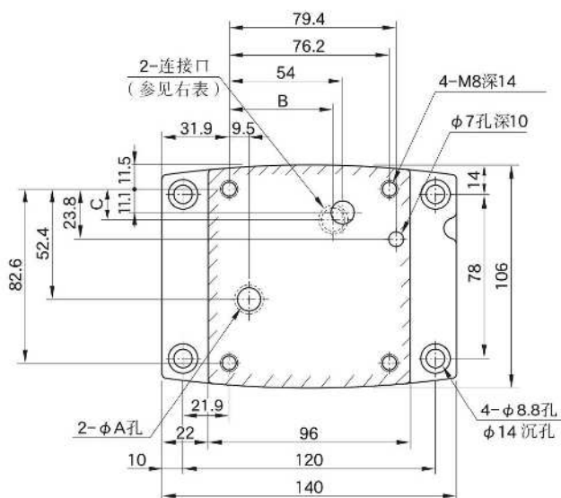
底板：FGM-03X, 03Y, 03Z
