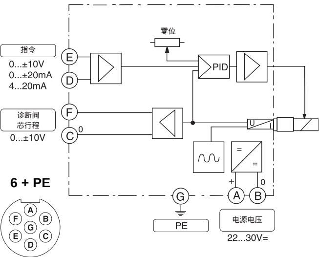
方框图 代号 0
