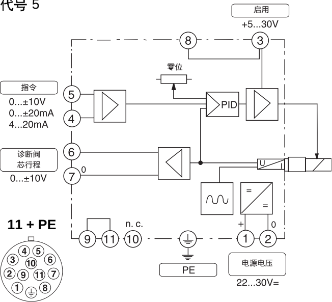
代号 5
