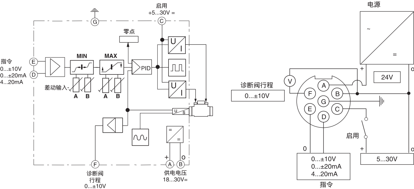
控制流程图, 阀电子控制器 接线
