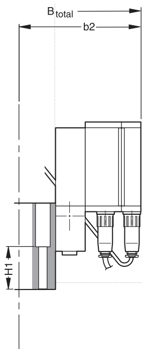
NG40 先导阀
