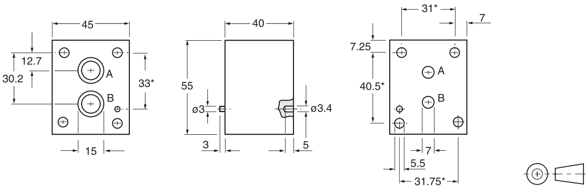
尺寸公差
