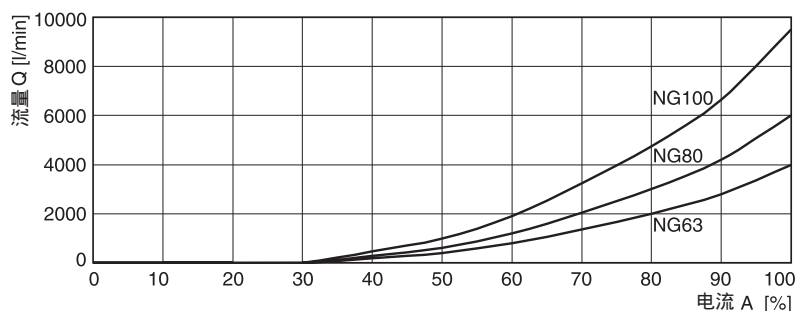
电磁铁电流/流量特性曲线 NG63-100 (Äp = 10 bar)
