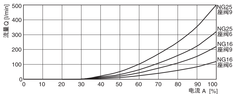
电磁铁电流/流量特性曲线 NG32-50 (Äp = 10 bar)
