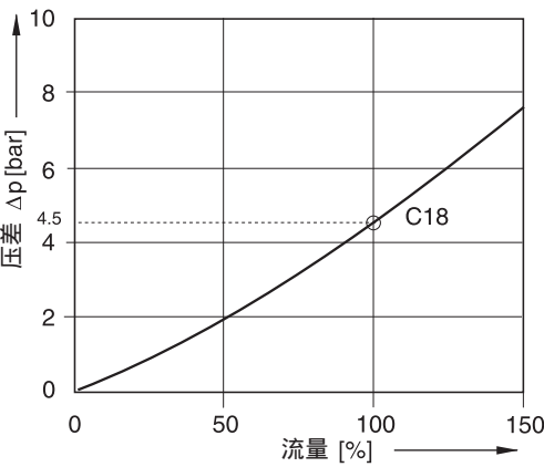
流量曲线
