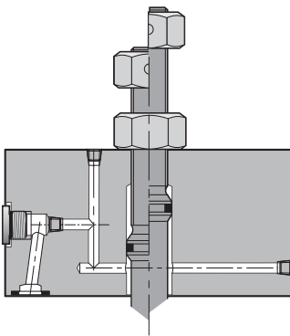
用于安装带有行程限制和带有"X"油口的液控系统,用在外控
