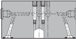
用于安装带有X,Y,Z1和Z2 的液控系统
