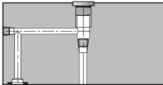
用于安装带有"X"油口的液控系统,用在外控
