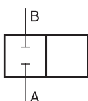
滑阀结构
