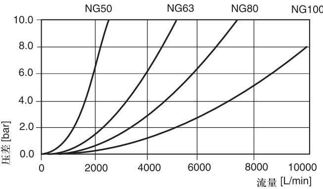
座阀芯 01, 04, 07
