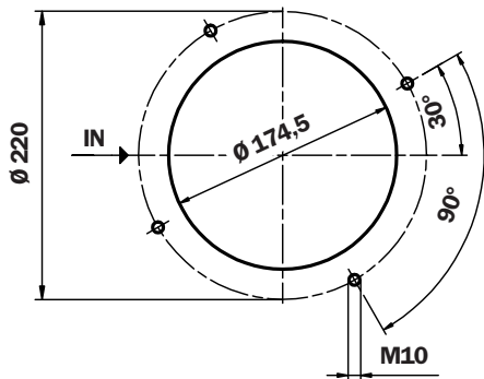
油箱上的孔
