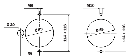
油箱上的孔 MPT 100/101
