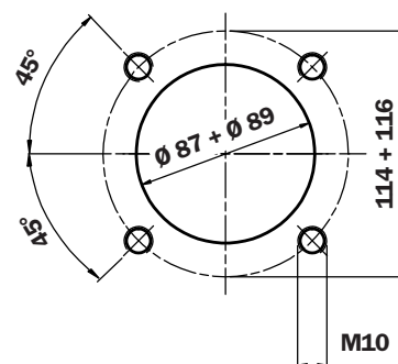
油箱上的孔
