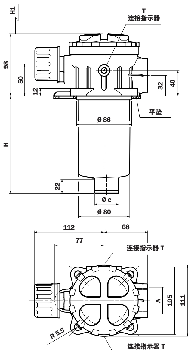
油箱上的孔
