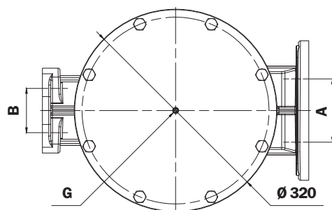
油箱上的孔
