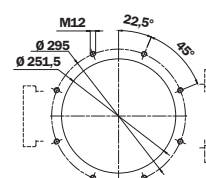
油箱上的孔
