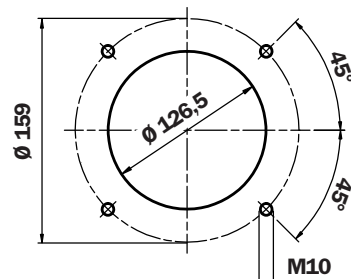
螺纹连接 MPF 184/194
