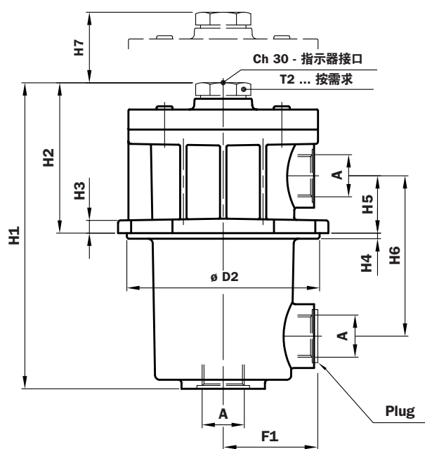
螺纹连接
