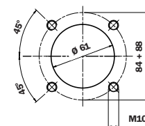
油箱上的孔 MPT 024
