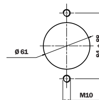
油箱上的孔 MPT 020/021
