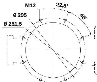
油箱上的孔
