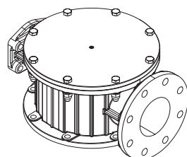
DN - SAE连接示意图
