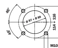
油箱上的孔 MPT 104
