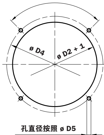
油箱上的孔 90°
