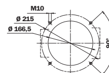
油箱上的孔
