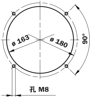
油箱上的孔
