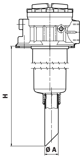
“H” 尺寸 装配有标准尼龙延长管的过滤器 (左侧a图)
