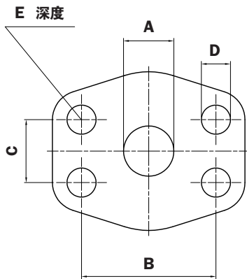
法兰 SAE 3000 PSI
