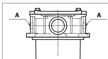
MPF 450/451
