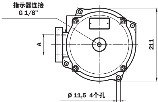
油箱上的孔
