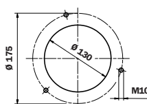
MPF 180
