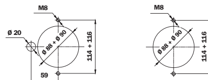
油箱上的孔
