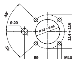
油箱上的孔 MPT 104
