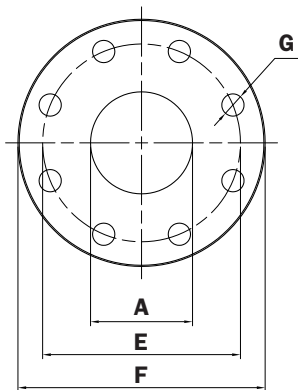
法兰 DN 100 PN 10/16
