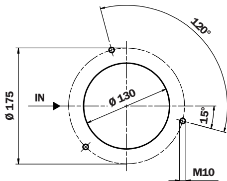
油箱上的孔
